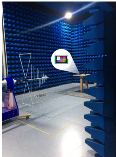
图 4-4 RE 测试图
