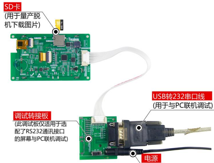
图 1-5 调试工具图
